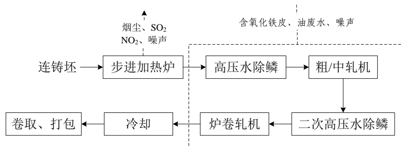
图3.2.1-16 不锈钢炉卷热轧生产工艺流程及产污节点
