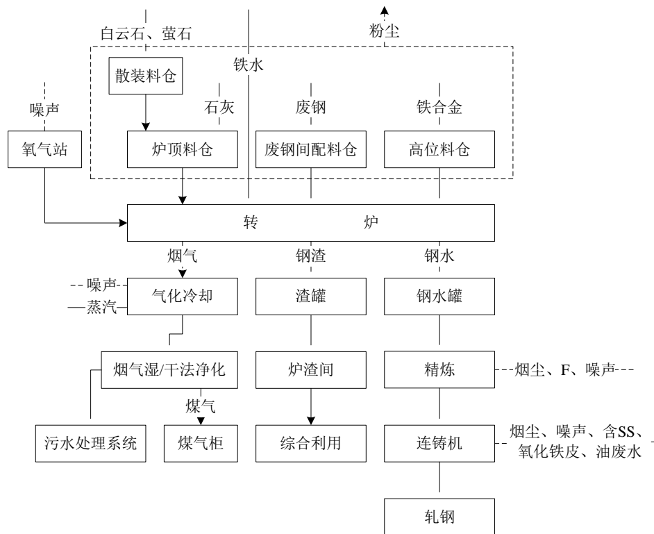
图3.2.1-13 碳钢炼钢生产工艺流程及产污节点
