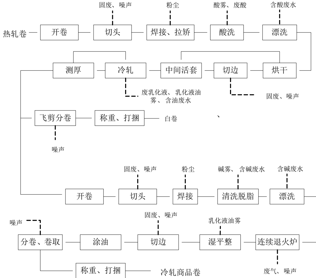
图3.2.1-17 酸洗、冷轧生产工艺流程及产污节点
