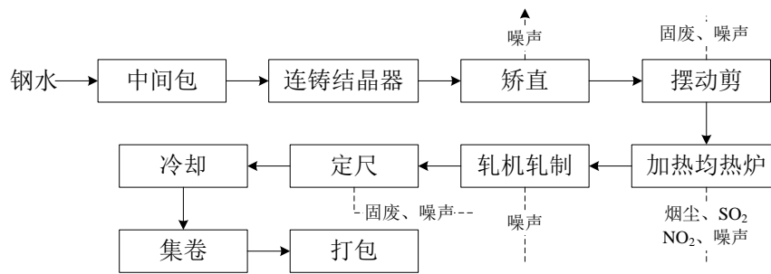
图3.2.1-15 2250mm热轧板生产工艺流程及产污节点
