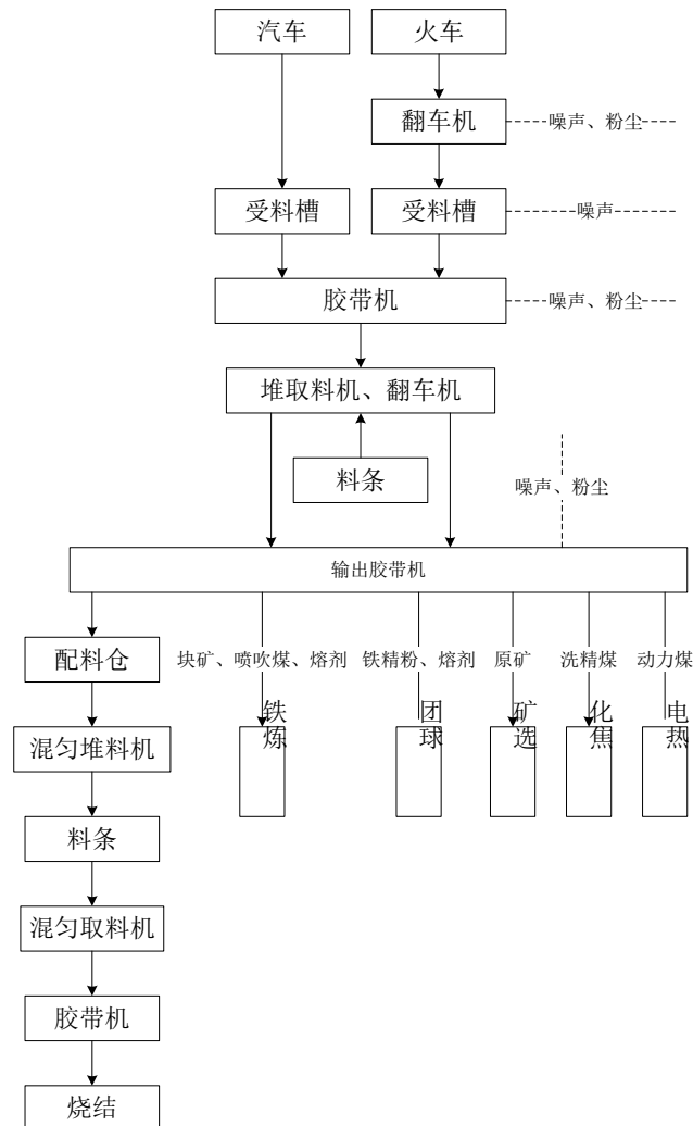
图3.2.1-1 原料场工艺流程及产污节点
