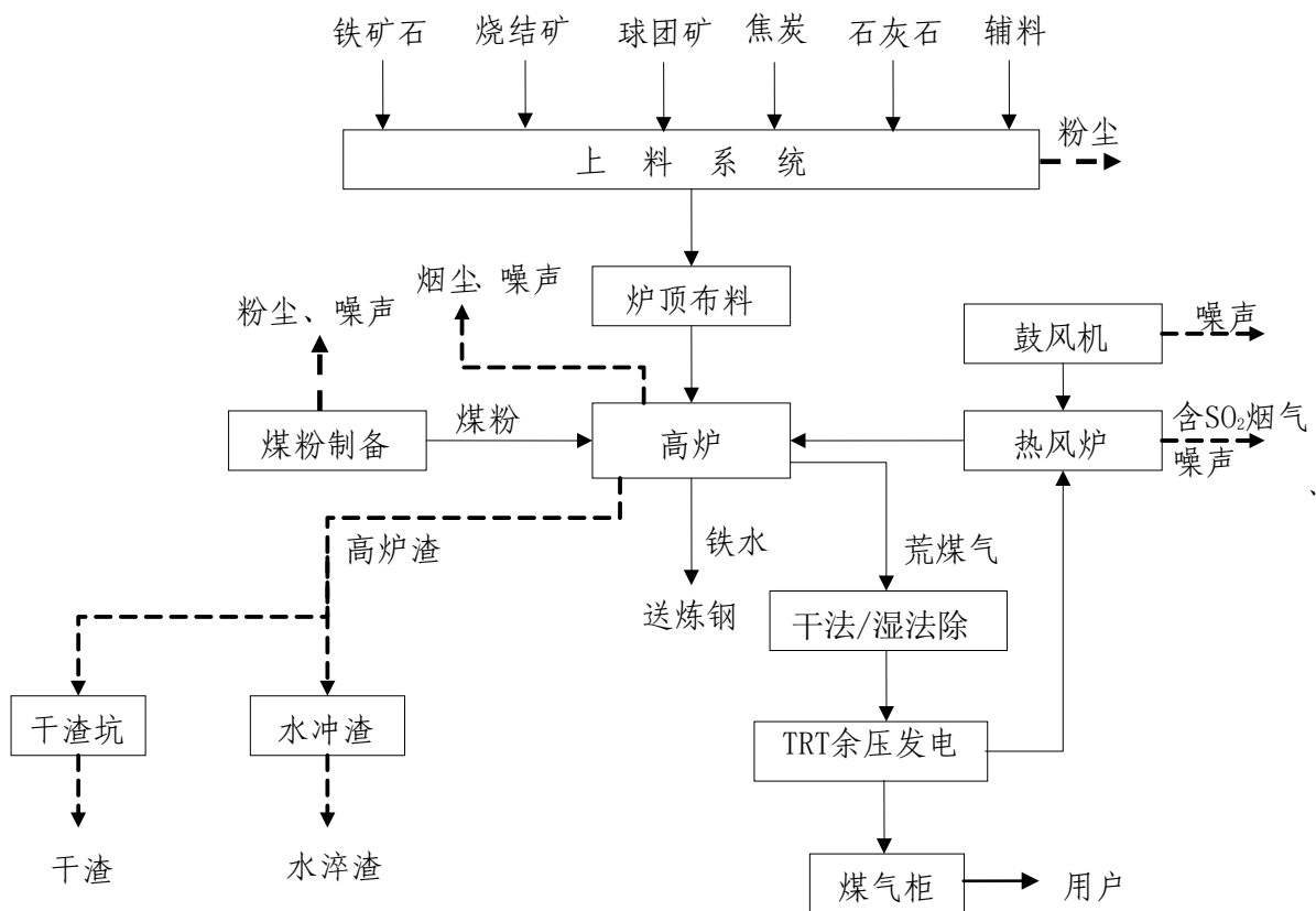
图3.2.1-12 炼铁生产工艺流程及排污节点
