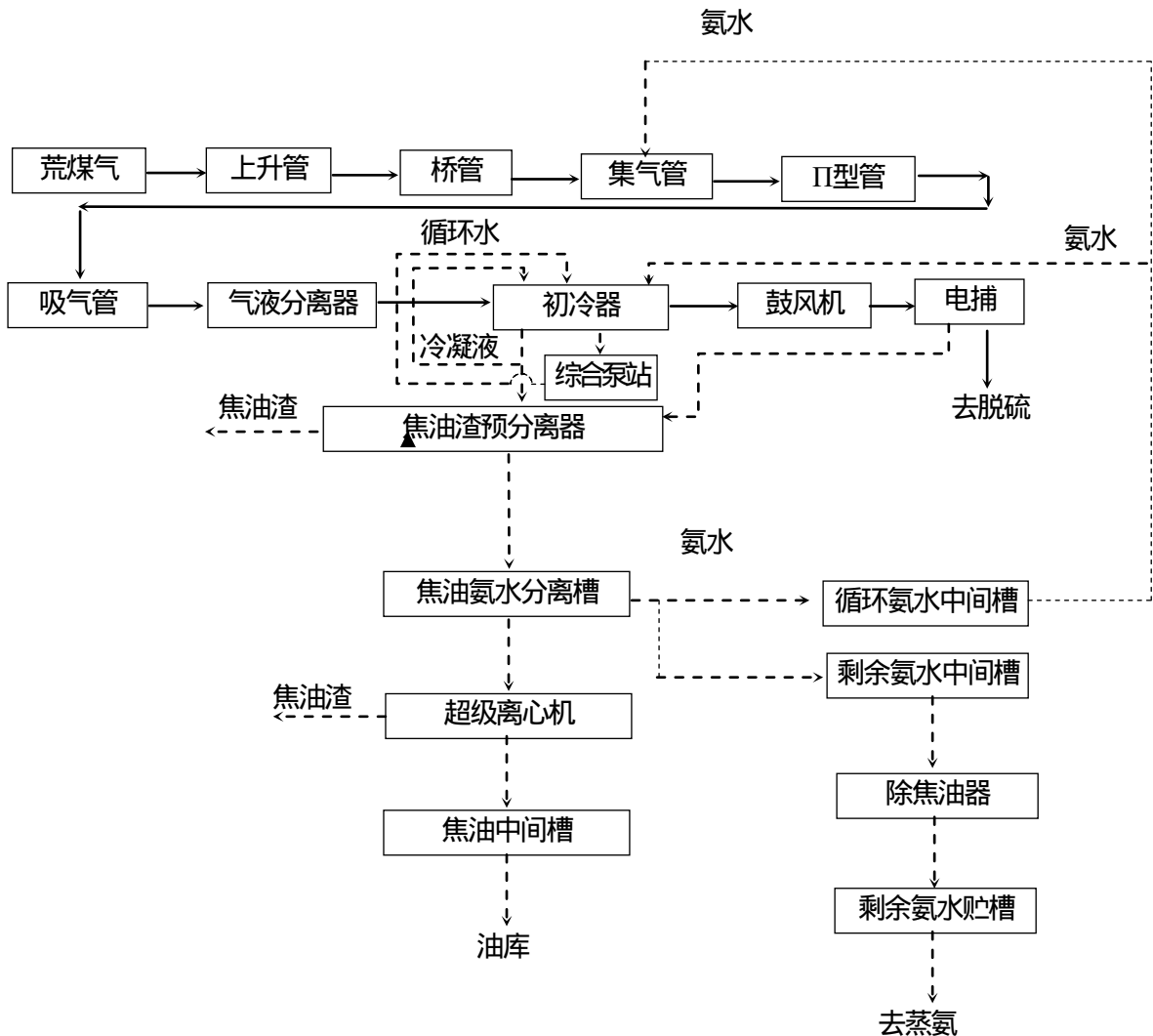
图 3.2.1-8 冷凝鼓风作业流程图
