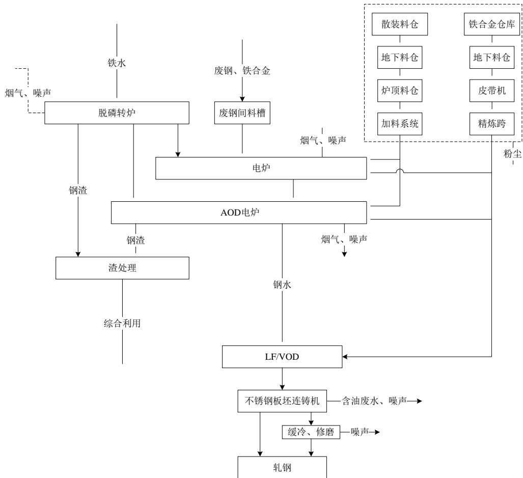
图3.2.1-13 300系不锈钢冶炼工艺流程及产污节点
