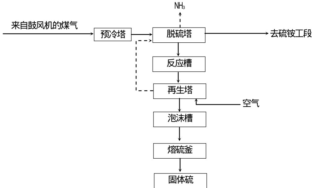
图 3.2.1-9 脱硫作业工艺流程及产污节点
