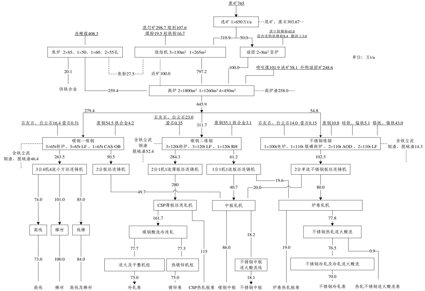
图3.1-1 物料流程图
