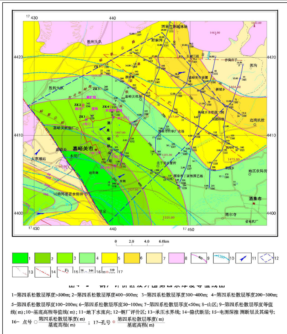
图3.3-2 区域第四系厚度等值线图
