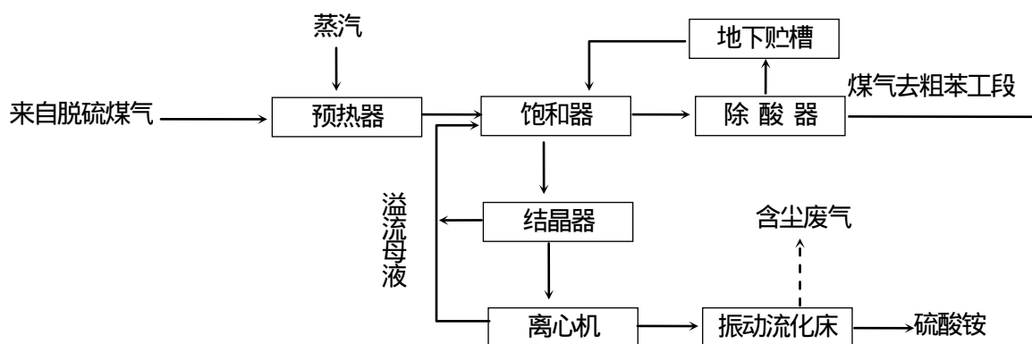
图 3.2.1-10 硫铵作业工艺流程及产污节点
