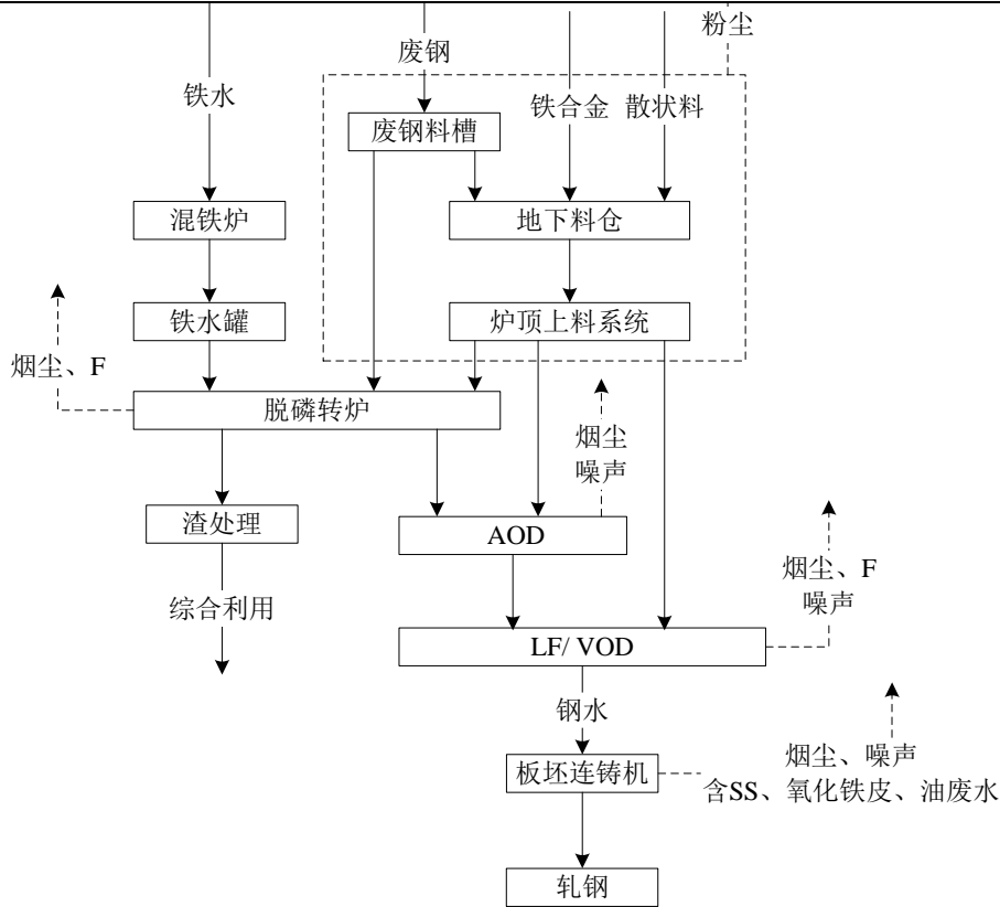
图3.2.1-14 400系不锈钢冶炼工艺流程及产污节点
