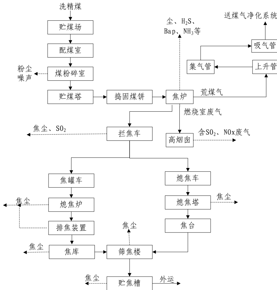
备煤、炼焦、干熄焦工艺流程及排污示意图 3.2.1-6。
