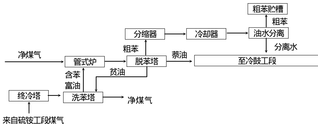
图 3.2.1-11 粗苯作业工艺流程
