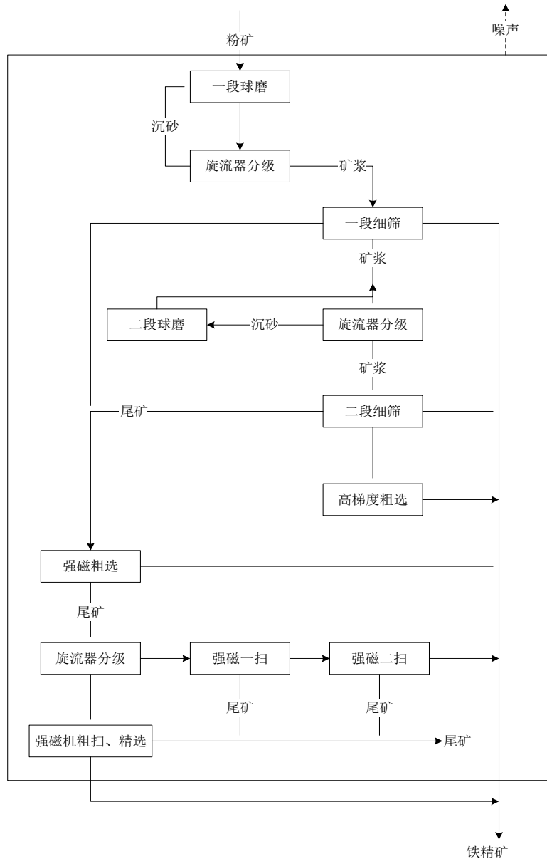
图3.2.1-3 强磁选工艺工艺流程及产污节点
