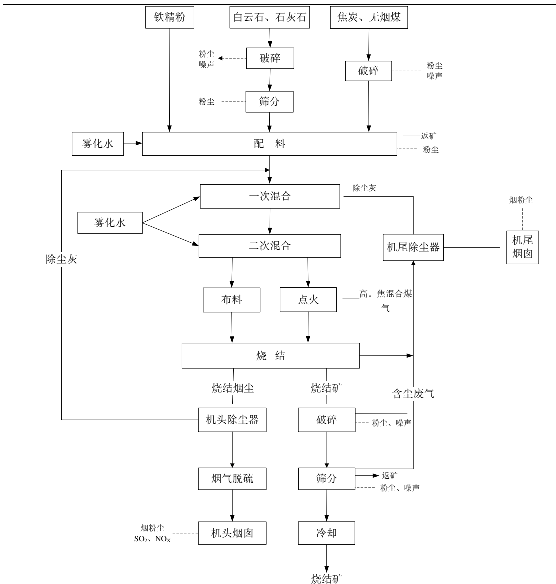
图3.2.1-5 烧结工艺流程及产污节点
