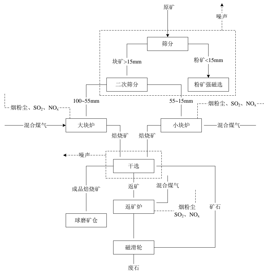
图3.2.1-2 原矿筛分及竖炉磁化焙烧工艺流程及产污节点
