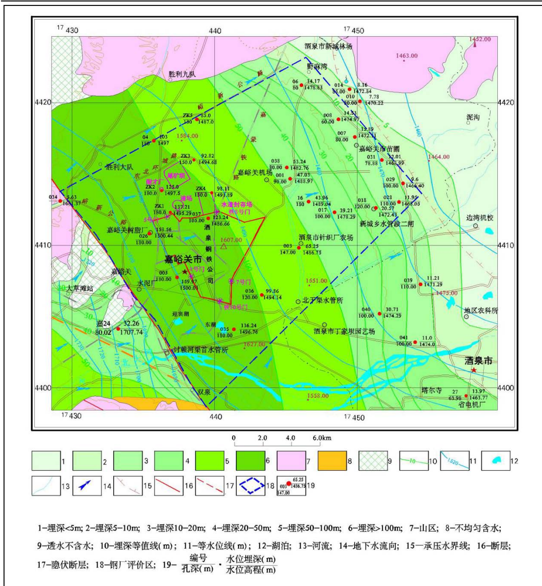
图3.3-7 区域潜水水位埋深及等水位线图
