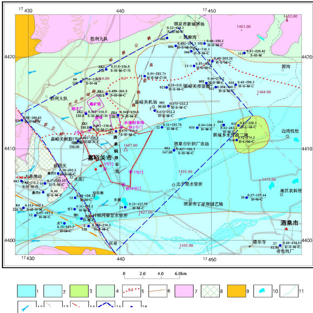
1-重碳酸盐类水; 2-重碳酸-硫酸盐类水; 3-重碳酸-氯盐类水; 4-硫酸盐类水; 5-矿化度等值线(g/l); 6-水化学类型界线; 7-山区; 8-古阶地; 9-不均匀含水; 10-水库; 11-河流; 12-地下水流向; 13-承压水界线; 14-隐伏断层; 15-钢厂评价区; 16-水化学分析点 编号· 矿化度(g/l)-总硬度(mg/l) 水化学类型
