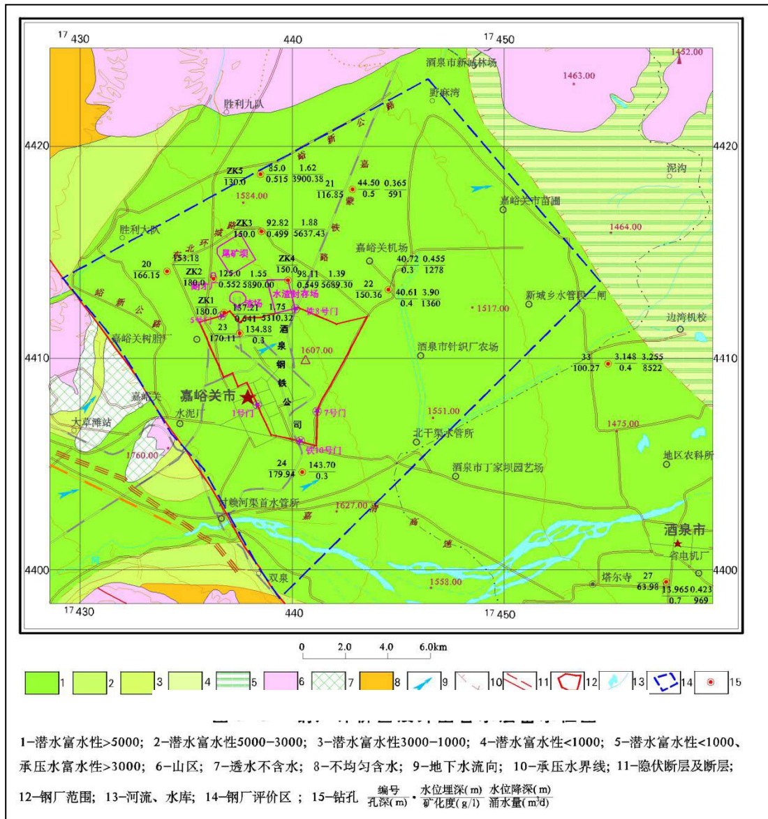
图3.3-6 区域含水层富水性图
