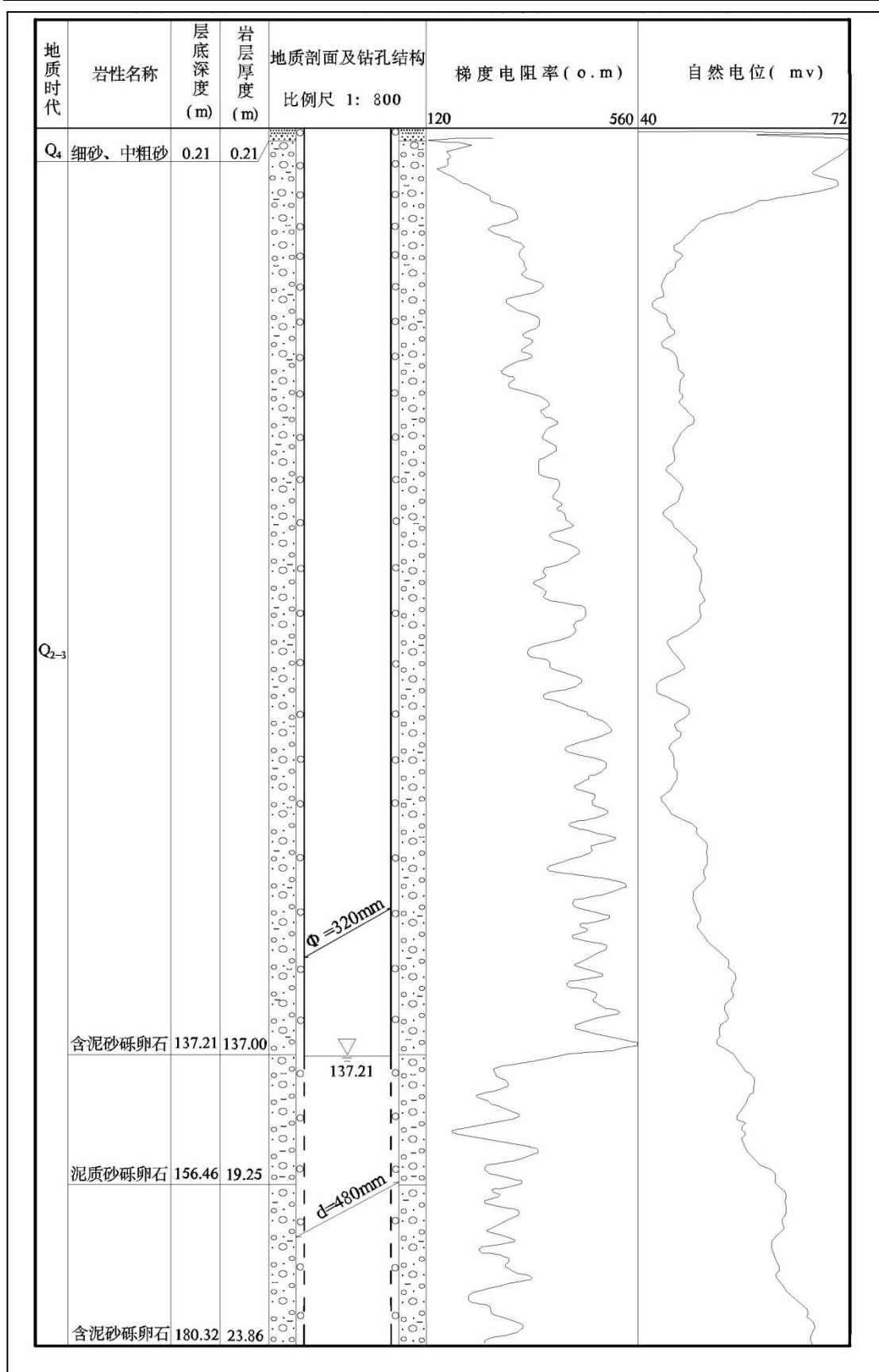
图3.3-4 ZK1号孔钻孔柱状剖面图
