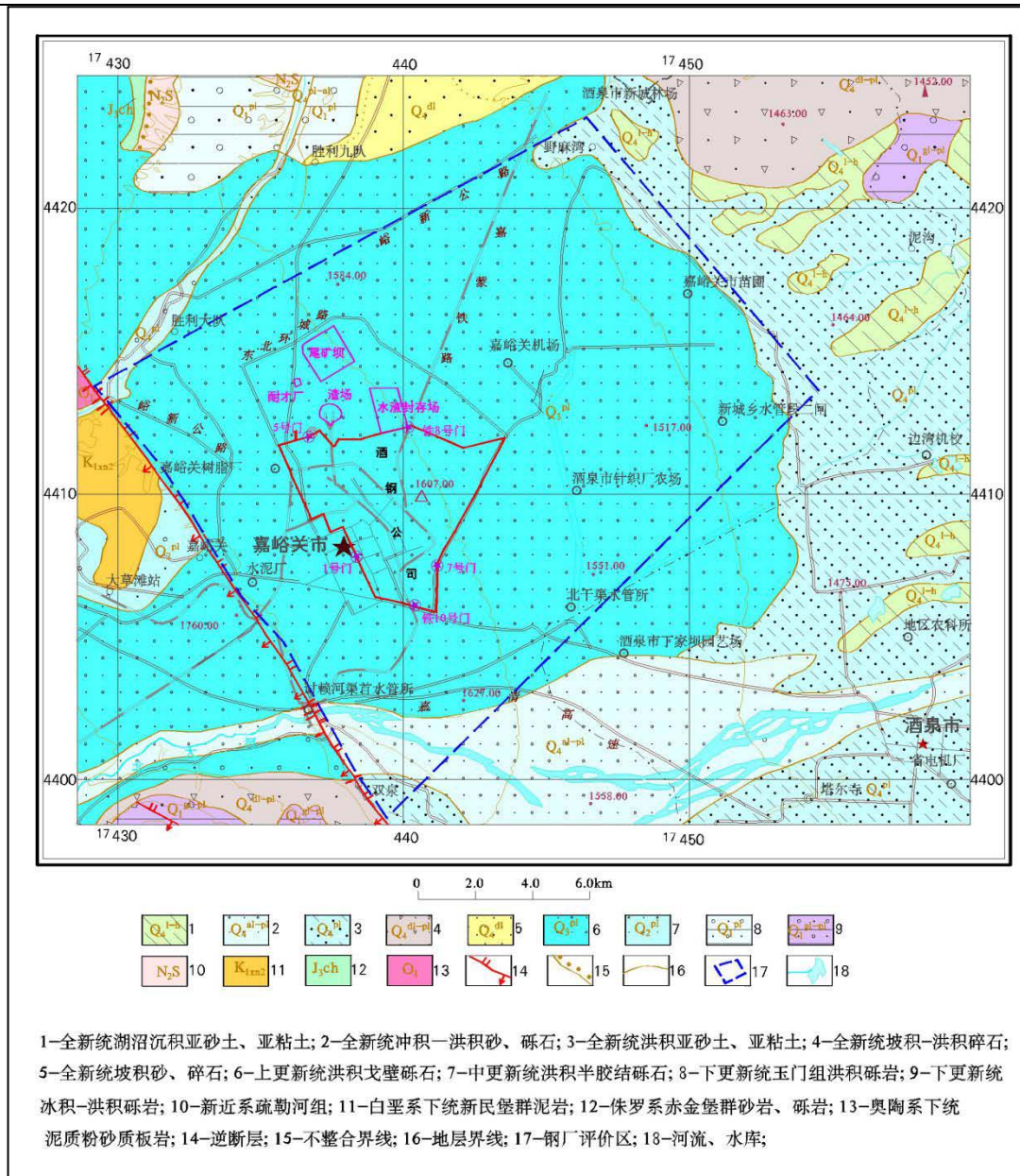
图3.3-1 区域地质图
