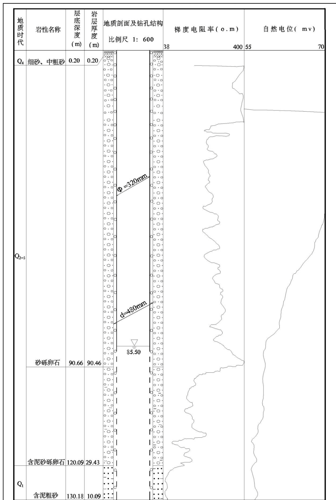
图3.3-5 ZK5号孔钻孔柱状剖面图
