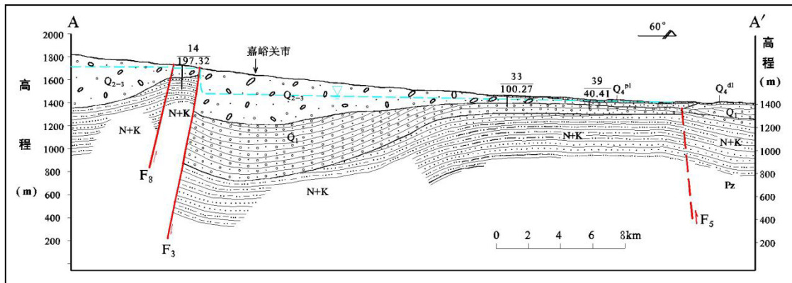
图3.3-3 区域水文地质剖面图
